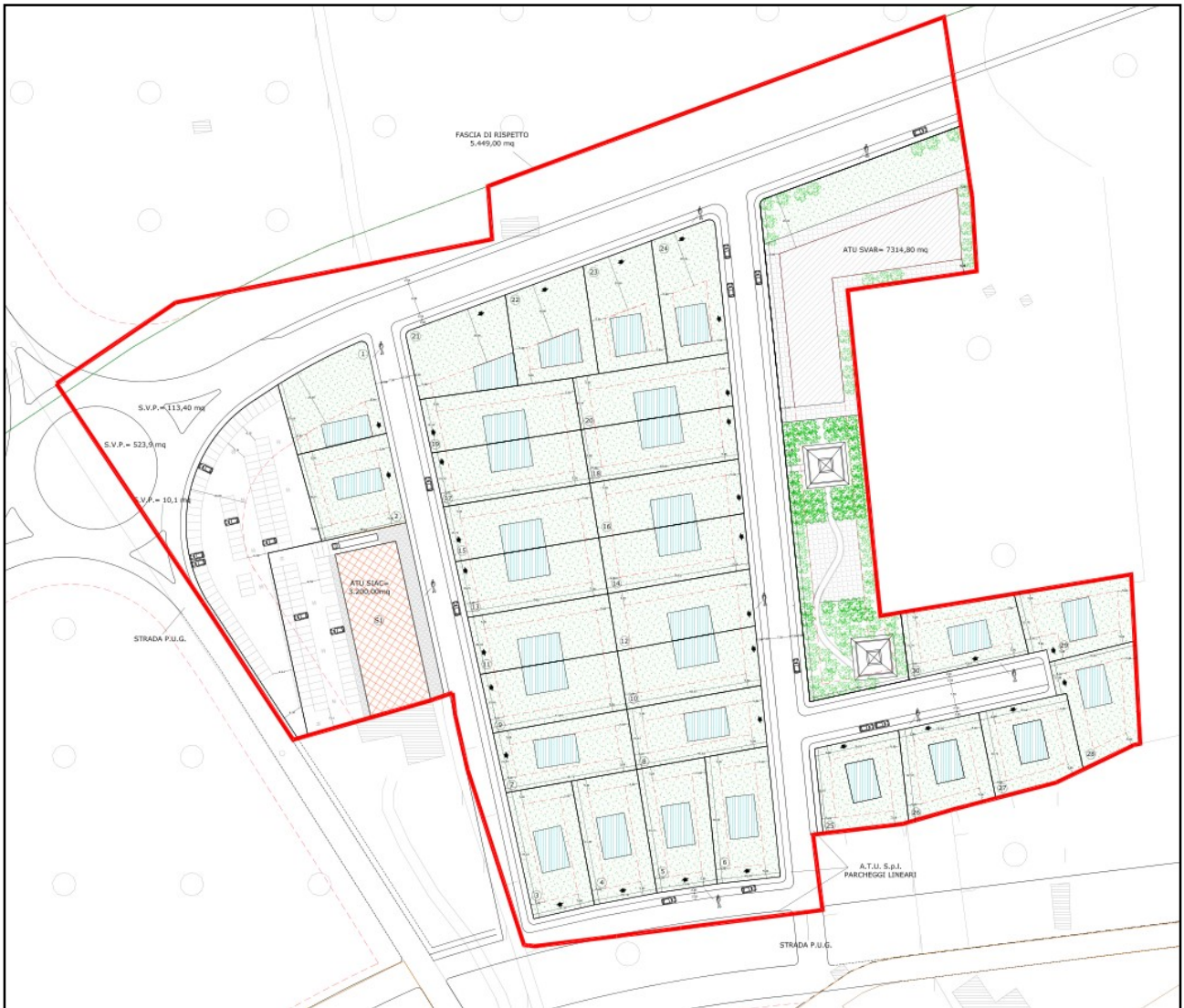
Figura 2 – Planimetria generale PUE adottato (rif. Tav. 004 Progetto 2014)
